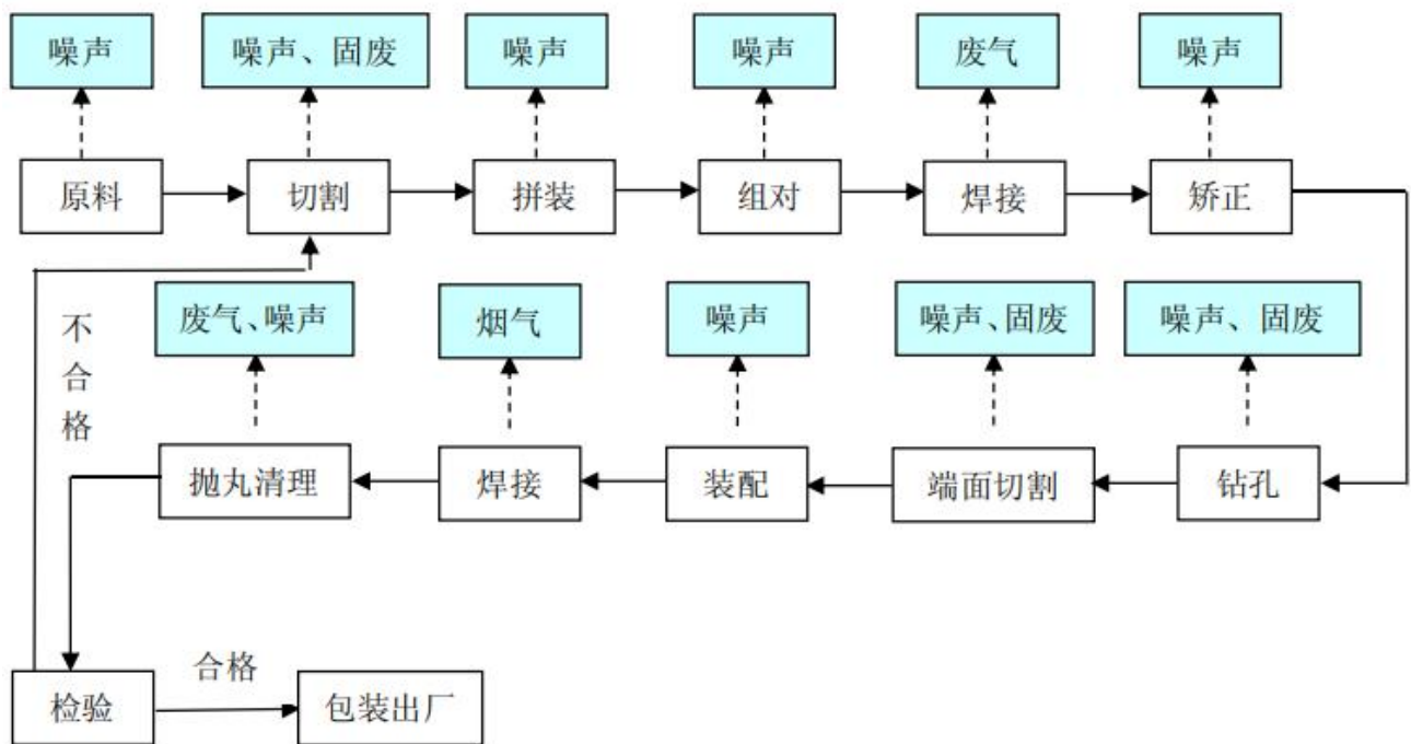
图 2-1 项目运营期工艺流程及产污图
